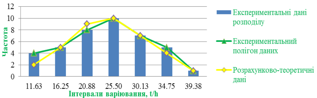
Рисунок 3.1 – Розподіл значень інтенсивності вхідного потоку вантажів за нормальним законом розподілу: ступінь вільності 4; рівень значущості 0.05; критичне значення критерію Пірсона 9.49; розрахункове значення критерію Пірсона 2.36
